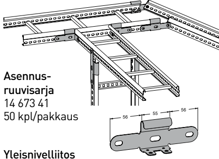
Yleisnivelliitos 14 670 18
