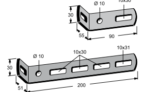
Asennusruuvisarja 14 673 41 50 kpl/pakkaus
