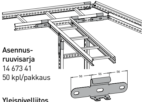
Yleisnivelliitos 14 670 18
