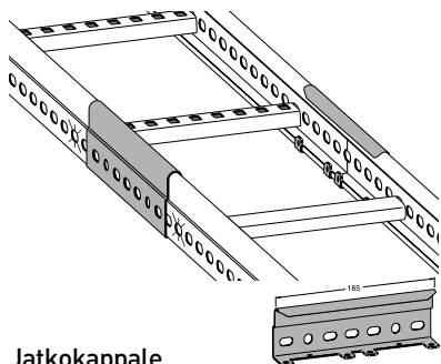
Jatkokappale 14 670 11
