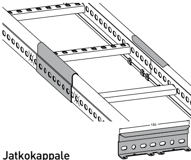
Jatkokappale 14 670 11
